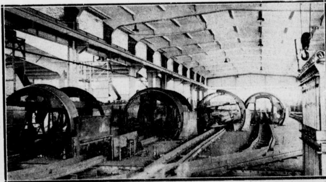
Abb. 2. Innere maschinelle Einrichtung
