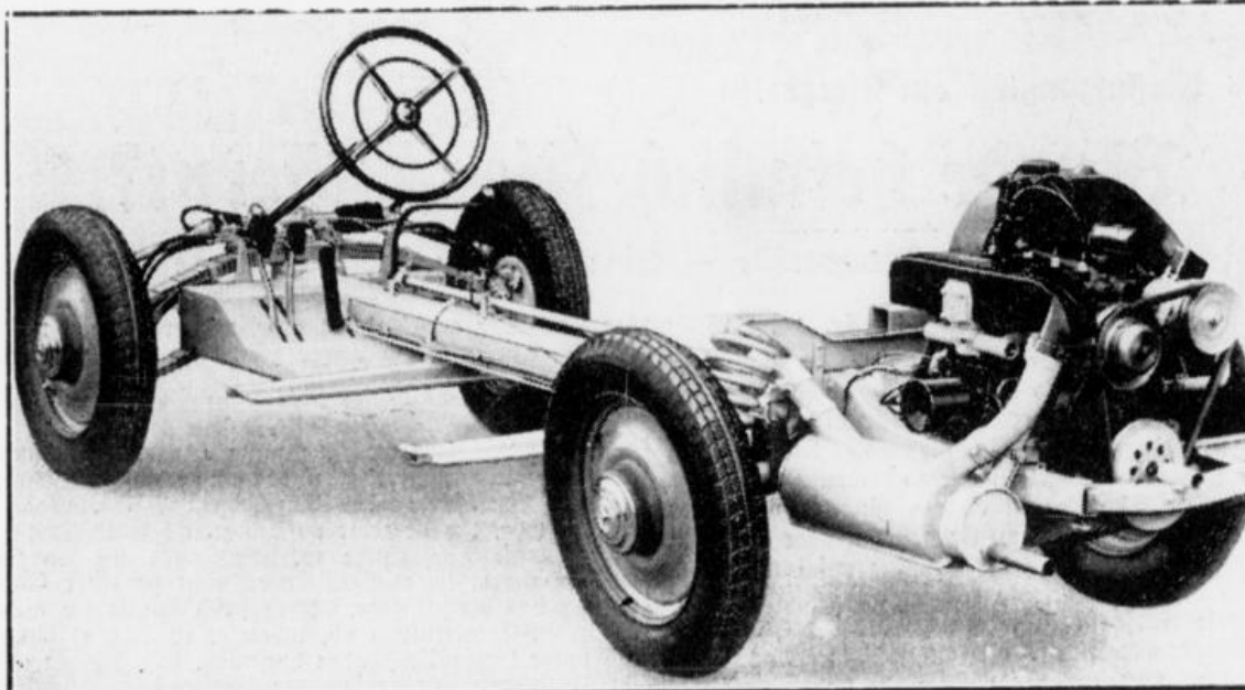
Fahrgestell des Mercedes-Benz-Heckmotorwagens Typ 170 V
