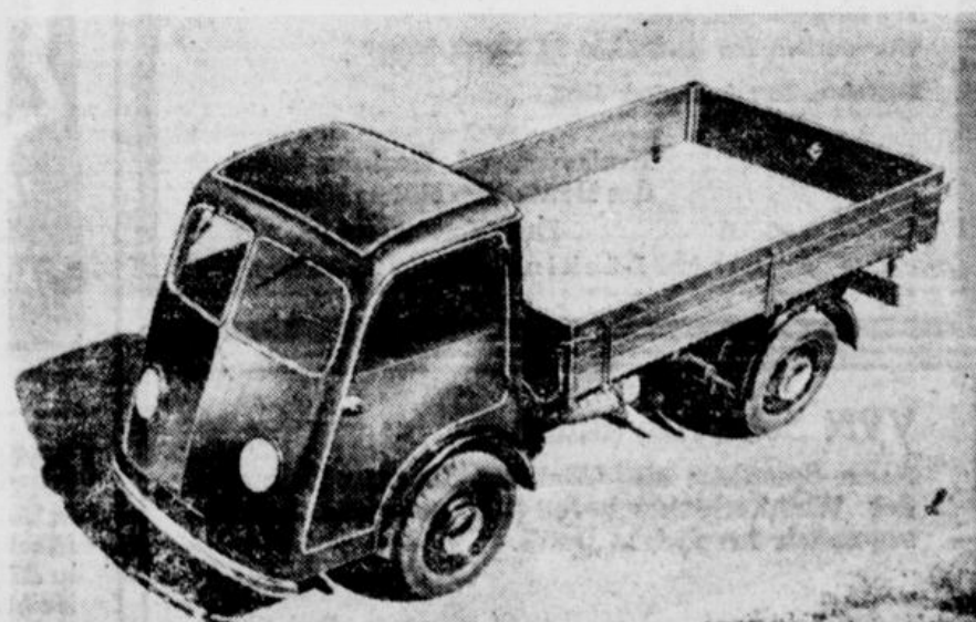
Ein neuer deutscher Kraftwagen, der 800 kg Nutzlast faßt ist der „Gutbrod Atlas 800“. Das Fahrzeug, dessen Höchstgeschwindigkeit bei 70 Stundenkilometern liegt, ist mit einem luftgekühlten Zweitakt-Heckmotor ausgerüstet, der 16,5 PS bei einem Treibstoffverbrauch von 7—9 Litern auf 100 km leistet.
