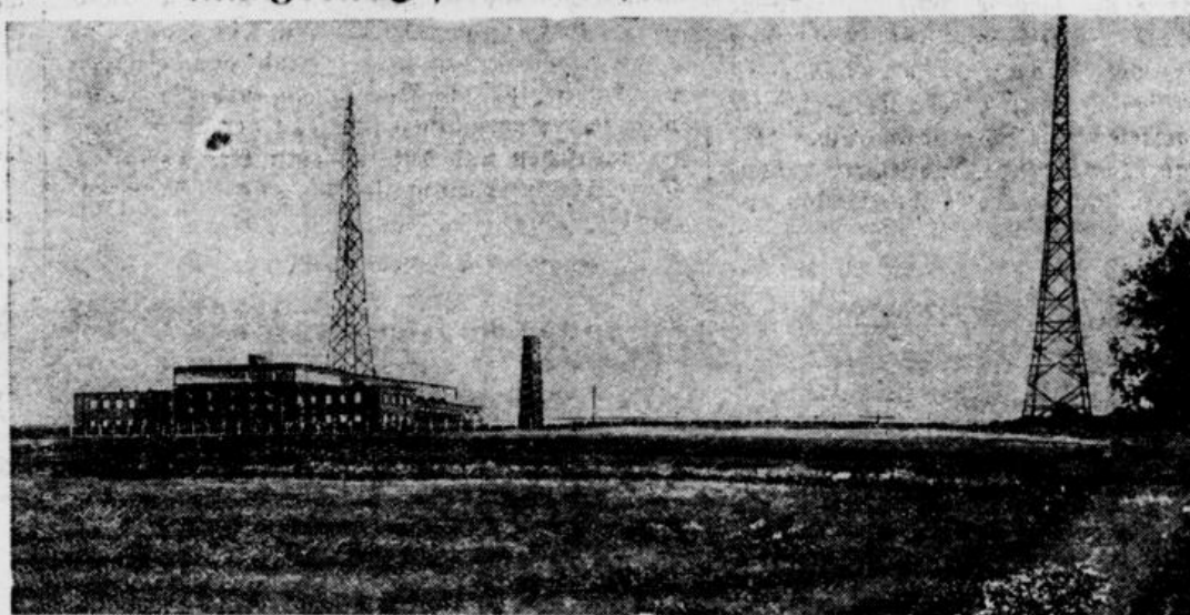
Der Groß-Rundfunksender Mülacker an der württembergisch-badischen Grenze. Er arbeitet mit einer Sende-Energie von 75 Kilowatt. Die Antennentürme sind 100 Meter hoch.
