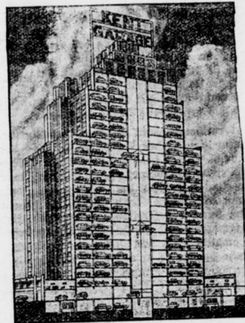
Garage: Schnitt durch eine Hochhausgarage (Reichsbahnhof, Leipzig). Der Mittelteil enthält eine Reihe von Schichten, die sich nach beiden Seiten hin öffnen lassen. Aus: „Der Große Brockhaus“, Bd. VI.
