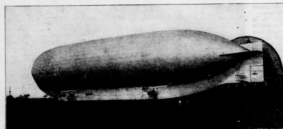
Das Stahlküstschiff V 1 des Ingenieurs Beh stellt den Versuch dar, die Vorzüge des starren mit denen des unfarren Systems unter Umgehung von beider Nachteilen zu verbinden. Auf der deutschen Luftschiffwerft G. m. b. H. erbaut führte das Luftschiff in den ersten Tagen des Juli in Düsseldorf seine gelungenen Probefahrten aus. Das 8000 Kubikmeter fassende halbbare Luftschiff ist zerlegbar, sein Traggerüst besteht vollständig aus Mannesmann-Stahlrohr, seine Länge beträgt 80 Meter, sein größter Durchmesser 13 Meter. In den beiden Gondeln, die durch einen mit einer Kabine versehenen Aufzug verbunden sind, befindet sich ein Daimlermotor von 130 PS. Die Gasbälle sind metallisiert. Als ein Vorzug des Ballons wird die leichte Entleerbarkeit durch Reißbahnen bezeichnet; dem Stahlgerüst, das feste Befestigung ermöglicht, sollen Stürme keine Gefahr bringen. Die konstruktiven Grundgedanken, die lebhaft an die Zeppelinluftschiffe erinnern, stammen von dem Ingenieur Beh, der das Luftschiff im Verein mit dem Flieger Dr. Wittenstein und dem Ingenieur Simon erbaut.
