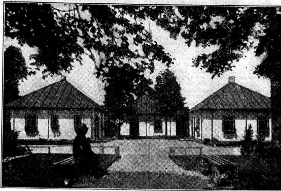
Die vereinigten Stahlwerke, Duisburg, haben Stahlhaus-Siedlungen bei Duisburg gebaut, deren kleine, schmale und farbenfrohe Häuser äußerlich von Steinbauten kaum zu unterscheiden sind. Bemerkenswert ist, dass sich die Mietpreise etwa auf die Hälfte der Mieten in steinernen Neubauten stellen.
