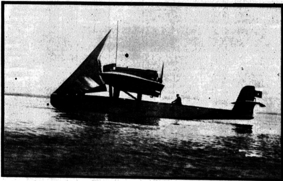
Der Dornier-Wal „Argus“. Die auf dem Bild gezeigte Besatzung ist für Notlandungen auf dem Meere vorgesehen. (Atlantic-Photo.)
