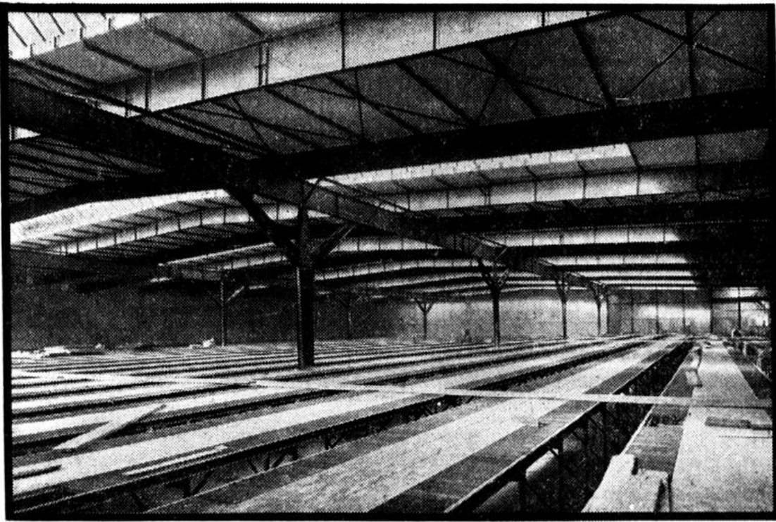
Einen gewaltigen Eindruck macht die 140 mal 80 Meter große Wagenhalle auf dem neuen Betriebsbahnhof der Bochum-Gelsenkirchener Straßenbahn an der Otto- und Wimmelhauser Straße in Bochum. Sie
