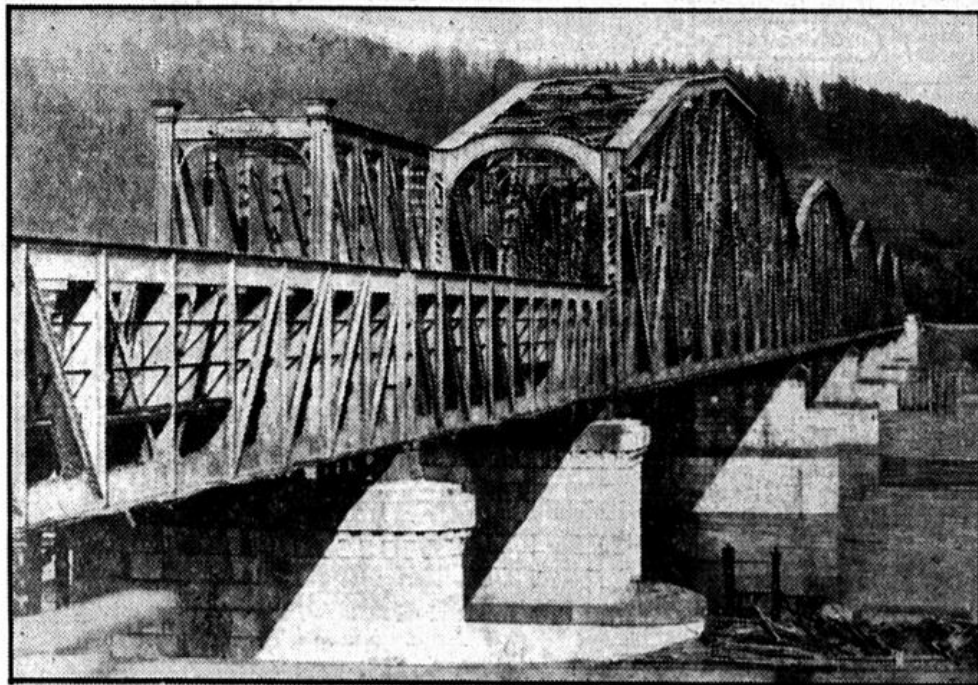
In Linz wurde vor kurzem die neue Donaubrücke dem Verkehr übergeben. (Atlantic Photo.)
