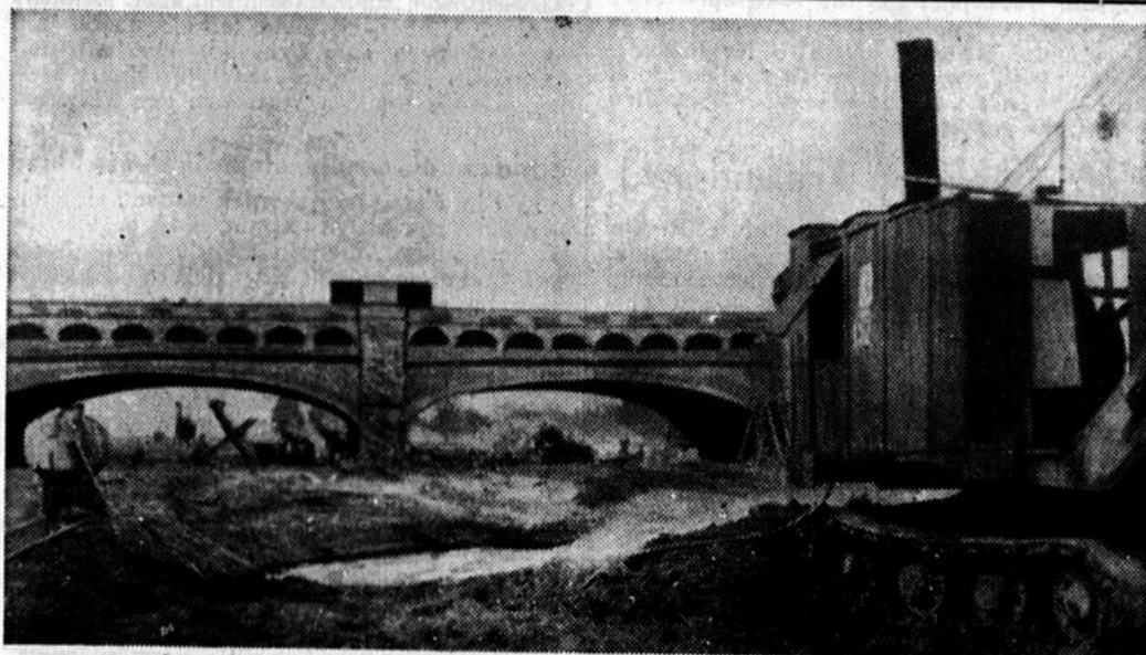
Zahlreiche Bagger bereiten der durch Trümmer versperren Weser ein neues Bett, welches unter einem anderen Brückenbogen der Kanalüberführung (auf unserem Bilde rechts) hindurchführen wird. Der zerstörte Teil des Aquadukts befindet sich weiter rechts.
