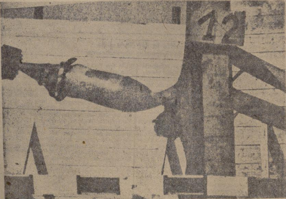
Die deutsche Waffentechnik ist dauernd bemüht, die Wirksamkeit unserer Bomben und Granaten durch laufende Verbesserungen zu steigern. Hier wird eine panzerbrechende Bombe geprüft. Der Vorgang wurde zum Teil mit der Zeitlupenkamera festgehalten. Auf dem Bilde links wird die Panzerbombe gegen das Prüfziel geschossen. Die Zeitlupenkamera hält den Einschußmoment im Bilde fest: Genau der
