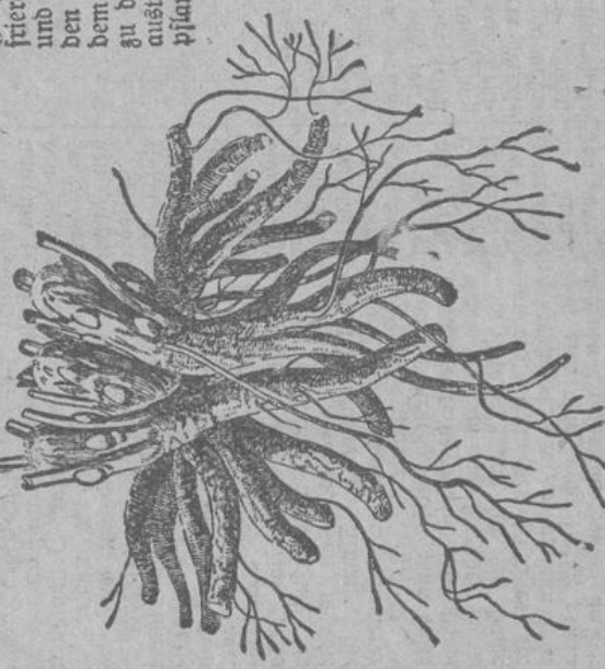
Abb. 2. Ein Pflanzling.
