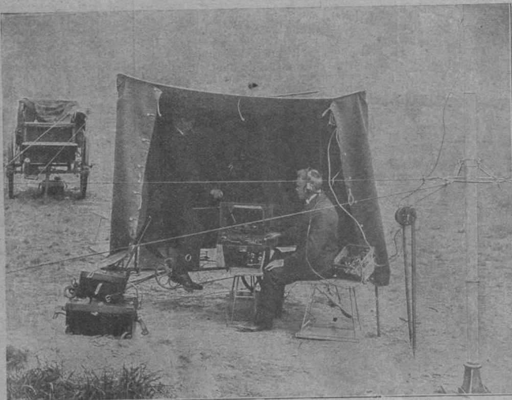
Die Telefunkenstation in Betrieb: Rechts die Auffangstange, unter dem Schutzbach der Telegraphist und die mit Fahrradtrieb ausgerüstete Dynamo-Maschine (Seite 387)
