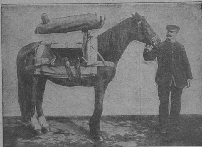
Die drahtlose Telegraphie und die Telefunkenstation in Naun: Eine in zwei Teile zerlegbare und zur Transportierung auf die beiden Pferde verteilte Telefunkenstation (Seite 387)
