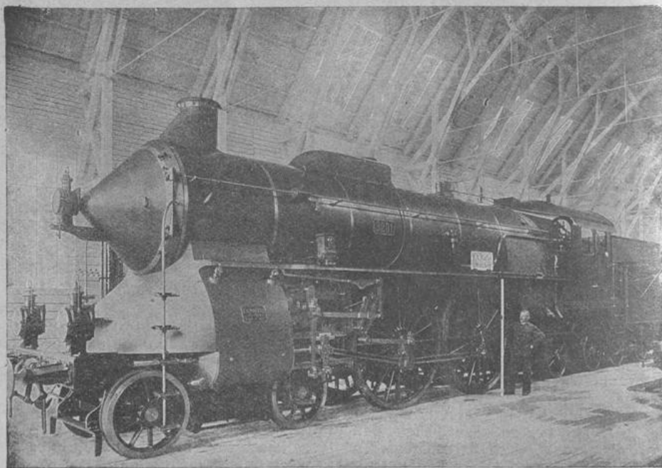
Die neueste Schnellzuglokomotive (Seite 310)
