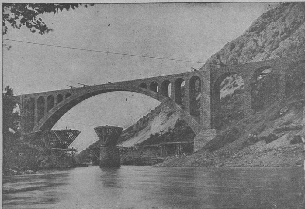
Im Bau begriffene Brücke über den Tsonzo (Seite 340)
