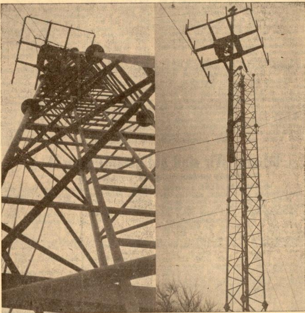
Die UKW-Station Nordhelle erhält einen zweiten Sender und dazu einen 65 Meter hohen Antennenmast. Unser Reporter erwischt einen Moment, in dem das Montagekommando auf das erste knappe Drittel der Masthöhe (20 Meter) eine große Plattform einbaut. Die Plattform ist mit einer Motorwinde hochgezogen worden und wird nun in die richtige Lage balanciert. (Fotos: Schulte)
