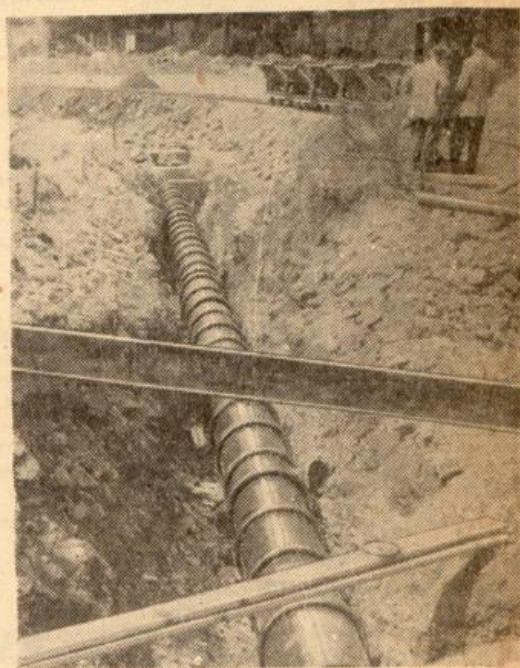
Die ersten 100 Meter der 1500 Meter lang werdenden Abwasserleitung sind bereits verlegt. Sie warten auf das Vergraben des Rohrmeisters. Dann wird der Schacht mit Hilfe der Feldbahn gleich wieder zugeschüttet.
