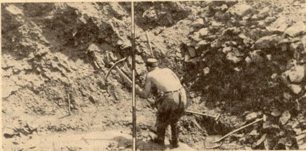
Hier buddelt man zwischen Felsen. So tief ist die Baugrube für das Schlammfangbecken im Rundkraterbecken ausgehoben worden. Grundwasser und Quellwasser sammeln sich an dieser tiefsten Stelle des Bauplatzes so stark, daß zwei elektrische Pumpen Tag und Nacht das Wasser aufsaugen müssen. Fotos: Conze
