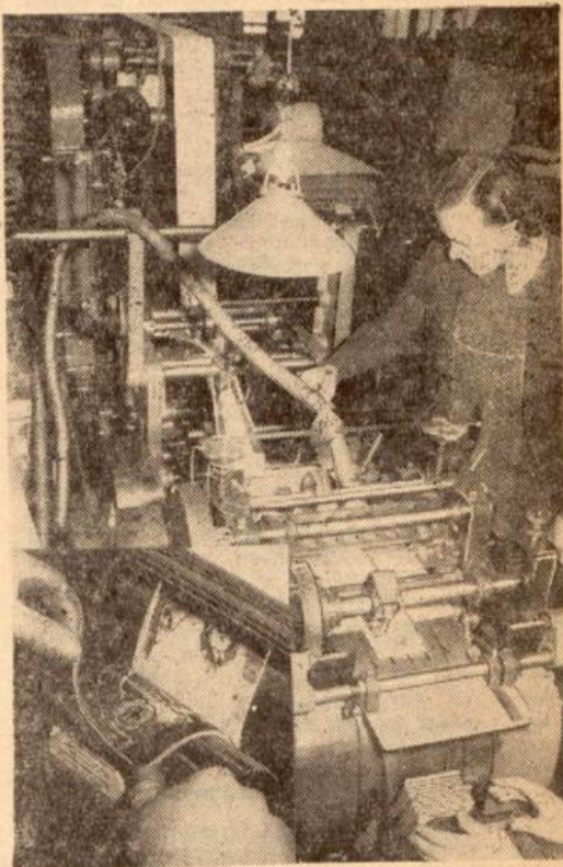
Blick auf die Beutelmaschine, die in einem Arbeitsgang aus dem Folienstreifen einen fertigen Beutel arbeitet. Der Streifen wird zunächst mit drei Farben bedruckt, dann geschnitten, gefalzt und schließlich geklebt. — Unten links: Das Gummi-Klischee wird noch einmal von der Walze gelöst, weil der Andruck gezeigt hat, daß die drei Farbdruke nicht haargenau aufeinander eingestellt sind. (Foto: Breitbach)
