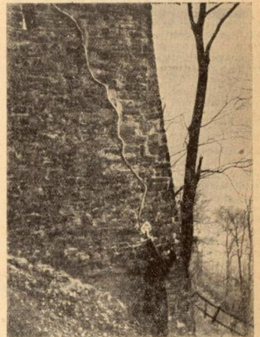
Ein Mauerriß in einem der Stützpfiler an der Westseite. Wenn das Mauerwerk, das durch den Riß abgetrennt wird, abrutschen sollte, würde es bis in die Stadt stürzen. Man erkennt, wie steil der Berg an dieser Stelle ist.
