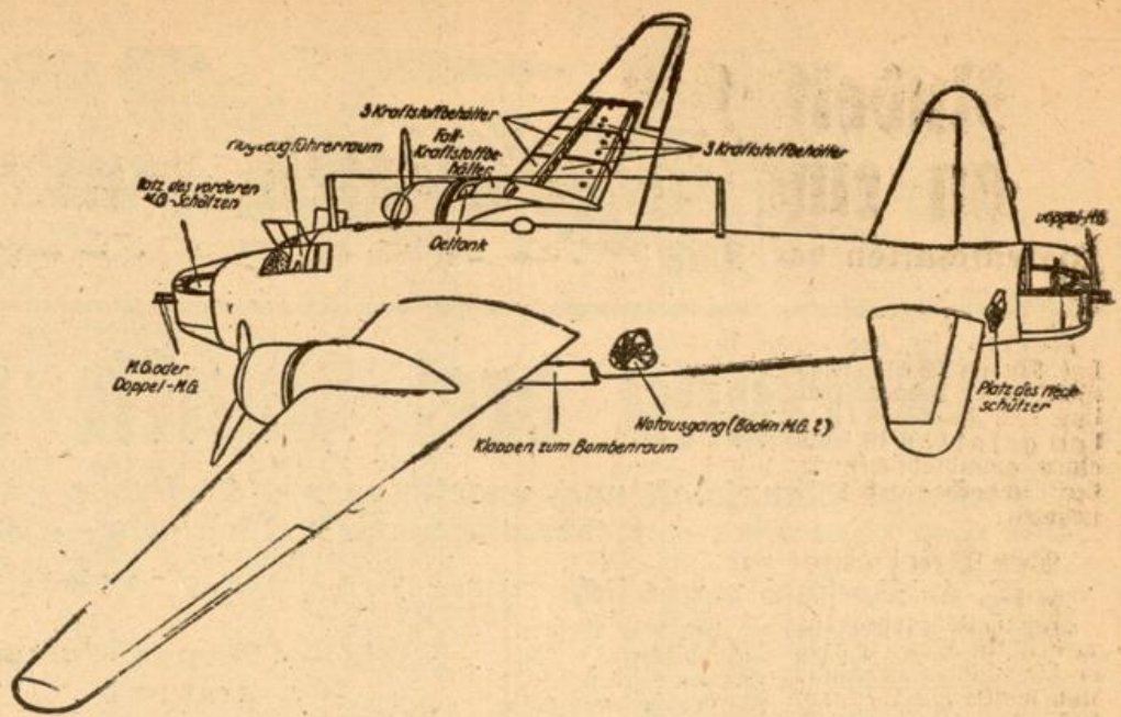
Von diesem Typ wurden bei der Luftschlacht über der Nordsee 36 Stück abgeschossen. Eine Zeichnung des britischen Kampfflugzeuges Vickers „Wellington“. Die Vickers-Wellington-Bomber gelten als die modernsten und besten englischen Maschinen. Weltbild (M).
