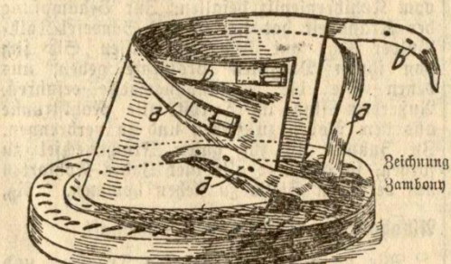
Abbildung 1 Pferdeschuh (Seitenansicht) a und b vergl. Text
