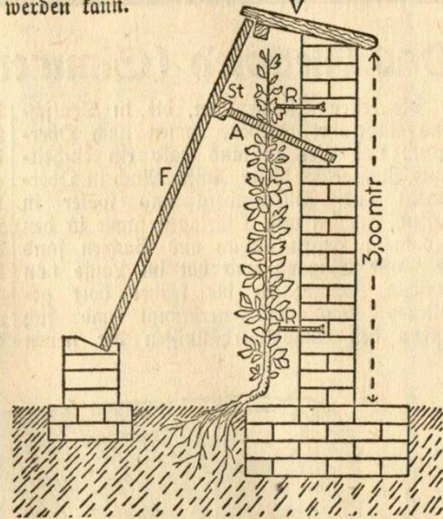
Glasfenster an der Obstmauer des Wohnhauses als Wetterstich A Eisenarm, F Glasfenster, R Rundstutzen, St Stützgerüst V Vordach
