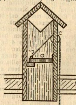
Einfacher Dunstschlot für den Stall
