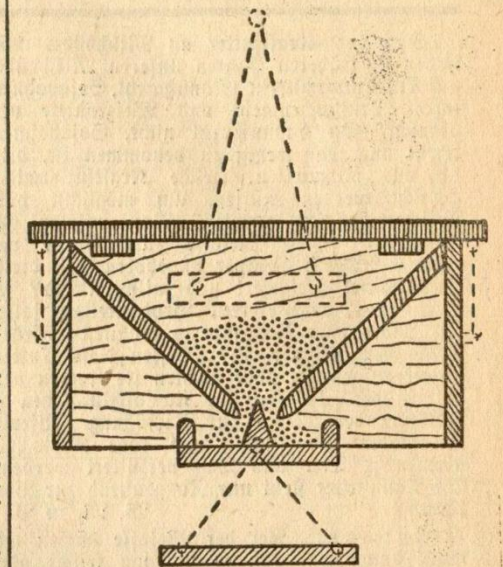
Abbildung 2 Futterkasten für Vögel (Querschnitt)
