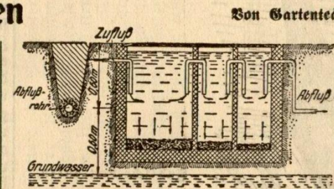
Abbildung 1. Klärgrube, im Dreikammersystem erbaut. In jeder Kammer findet selbsttätig die Klärung statt. Das geklärte Abwasser fließt in die Rohrleitung (links), die in einer Tiefe von etwa 60 cm verlegt ist.
