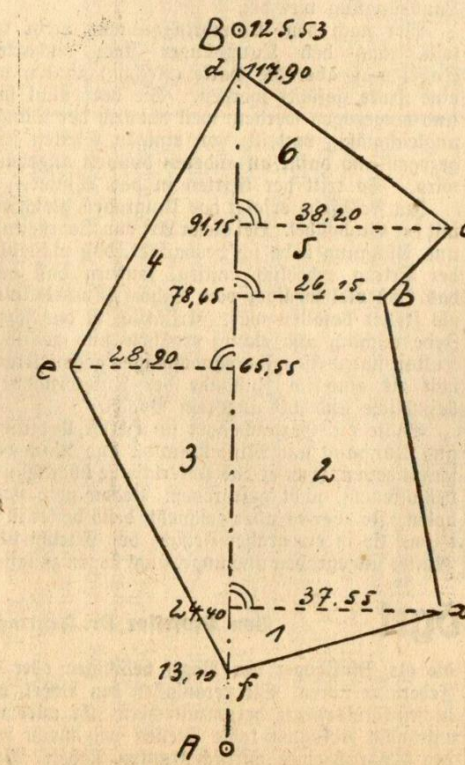
Abbildung 1. Messung und Berechnung eines gradlinig begrenzten Feldteiles (Vieleck).
