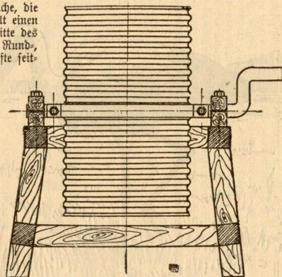
Abbildung 2 Querschnitt der auf einen Holzblock aufmontierten Beiztrommel
