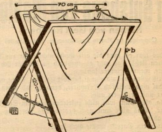
Klappbarer Sackaufhalter.
