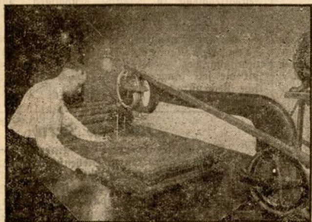
Die Bandmesser-Zuschneide-Maschine schneidet in einem Arbeitsgang bis zu 18 Lagen. Leistung in der 48-Stunden-Woche 900 Anzüge oder Mäntel.
