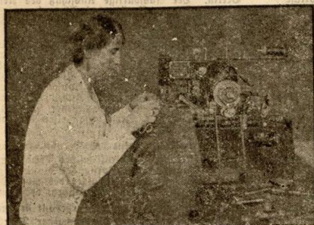
Die Reece-Knopfloch-Maschine, ein Wunderwerk der Technik. Leistung in der 48-Stunden-Woche 7000 Knopflöcher.
