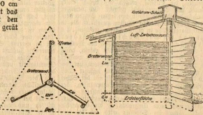
Abbildung 2. Viehschuppen, a Grundriss, b Querschnitt.
