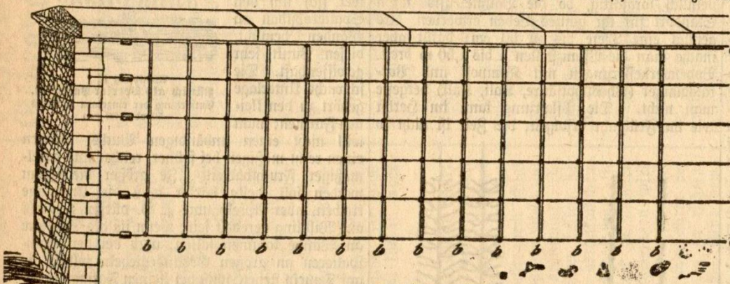
Abbildung 7 Anbringen eines Spalliergerüsts. a verzinkte Eisenbrücke (Entfernung voneinander 50 bis 100 cm). b Spallierlaten oder Längslatten (Entfernung 40, 50 oder 60 cm).
