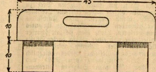
Abbildung 2. Obsthorden (Seitenansicht).
