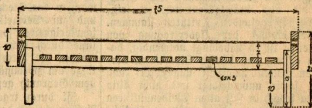
Abbildung 3. Obsthorden (Längsschnitt).
