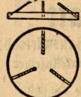
Abbildung 6. Querschnitt der Walzenreifen mit den drei Flacheisenbändern.
