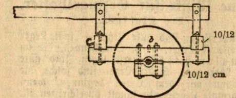
Abbildung 2. Seitenansicht.
