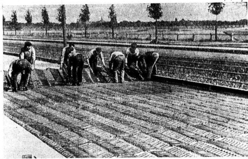
In Düsseldorf wurde mit dem Bau einer eisernen Straße begonnen, der ersten ihrer Art in Deutschland. Es gelang ein zickzackförmiger Stahlrost zur Verwendung, der in eine Teermischung eingebettet wird.
