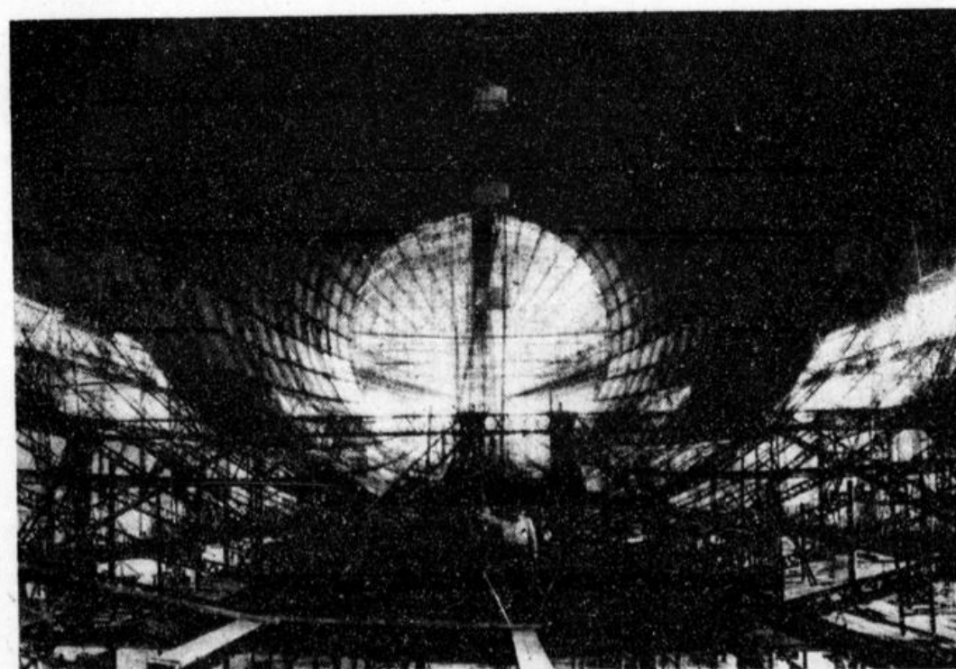
„Q3. 130“ fährt mit Helium Nachdem die Vereinigten Staaten von Nordamerika die Ausfuhr von Helium bewilligt haben, wird „Q3. 130“ für den Gebrauch von Helium eingerichtet. Unser Bild zeigt einen Blick in das Schiff nach dem Heck zu. Deutlich erkennt man die gewaltigen Ausmaße des Luftriesen. (Weltbild-M.)
