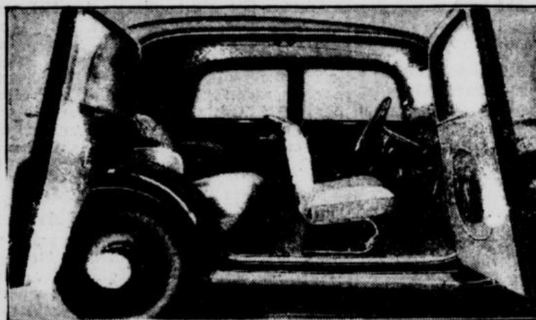
Der neue 4zylinder 1,4-Liter-30-PS-Stöwer; Vortrieb-Limousine ohne Mittelposten und Schwingachsen.
