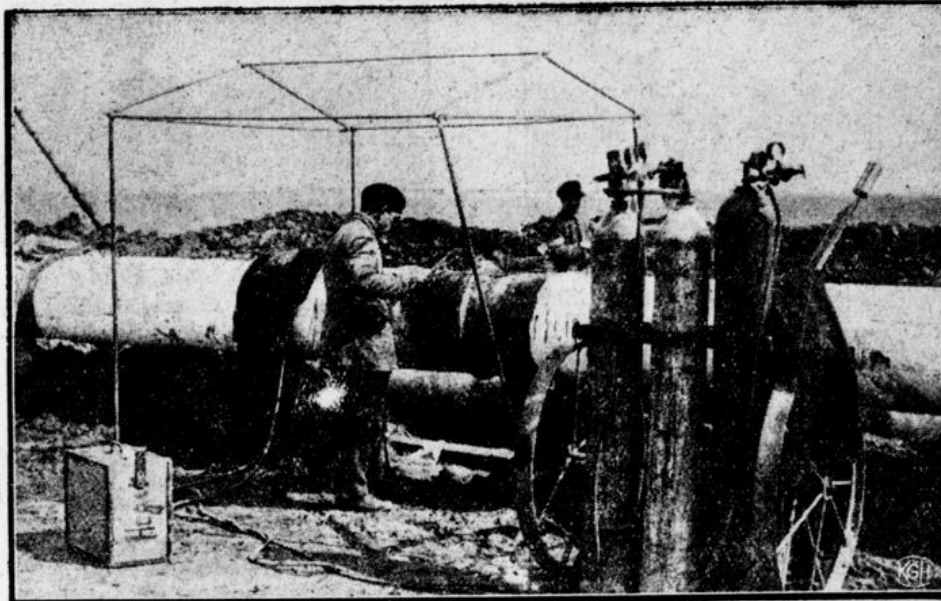
Schweißung zweier Rohrenden
