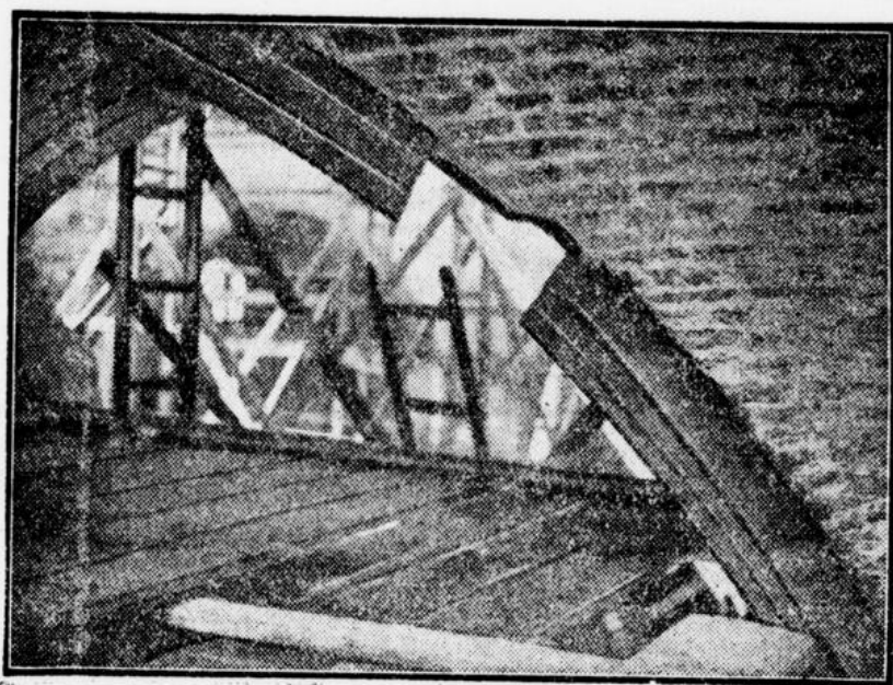
Unteres Bild: Bruchstelle im Maßwerk der Gewölbe. Rechtes Bild: Ein stark beschädigter Pfeiler nach der Reinigung.
