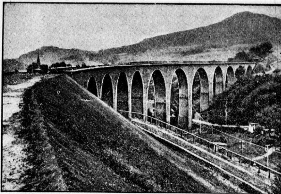
Bild links: Ein neues Meisterwerk deutscher Technik Deutschlands zweitgrößter Eisenbahnviadukt wurde vor kurzem an der Reichsbahn-Neubaustrecke Türkismühle-Musel, die das Grenzgebiet zwischen dem südlichen Rheinland, der Pfalz und dem Saarland erschließt, vollendet. Die große Talbrücke bei Oberkirchen (Bezirk Trier) ist 300 Meter lang, 38 Meter hoch und hat 12 Brückenbögen bis zu 25 Metern lichter Weite.
