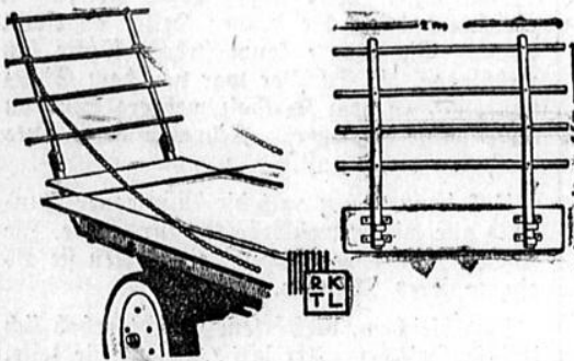
Der untere Teil der Stützen muß dabei natürlich aus Stahlprofilen, am besten U-Eisen, hergestellt sein. Sie lassen sich dann in Dosen an den Längsträgern unter der Plattform leicht
