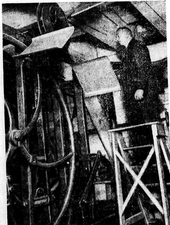
Das Spielwerk. Links das große Schwungrad; links oben das kleine Flügelrad mit den Flügeln, die für einen gleichmäßigen Lauf des Spielwerkes Sorge tragen.
