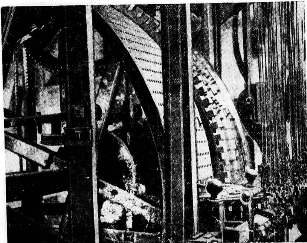
Die riesige Trommel, auf der mit Bronzeflöhen die Melodien des Glockenspiels eingegraben sind. Rechts das Gewirr der Drähte, die den Zug des Walzwerkes auf die Glocken übertragen.
