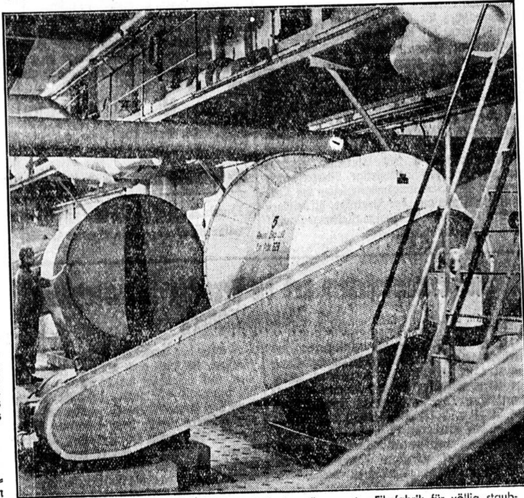
Eine riesige Klimaanlage sorgt in den Fabrikationsräumen der Filmfabrik für völlig staubfreie Luft von ständig gleichem Wärme- und Feuchtigkeitsgehalt
