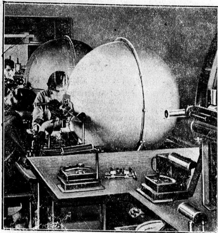
Güteprüfung durch das Kugelphotometer, das unbestechliche Maßgerät für die Prüfung der Lichtleistung
