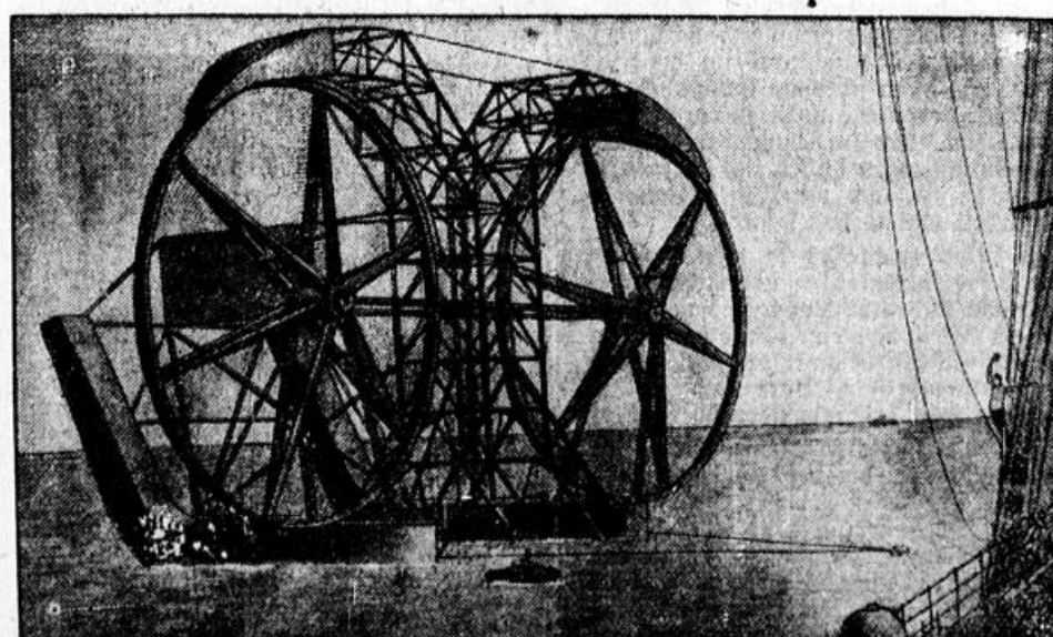
Eine auf Pontons aufmontierte Kraftwind-Apparatur.
