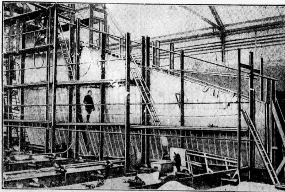
Der gewaltige Flügel des neuen Junkers-Flugzeuges im Bau.
