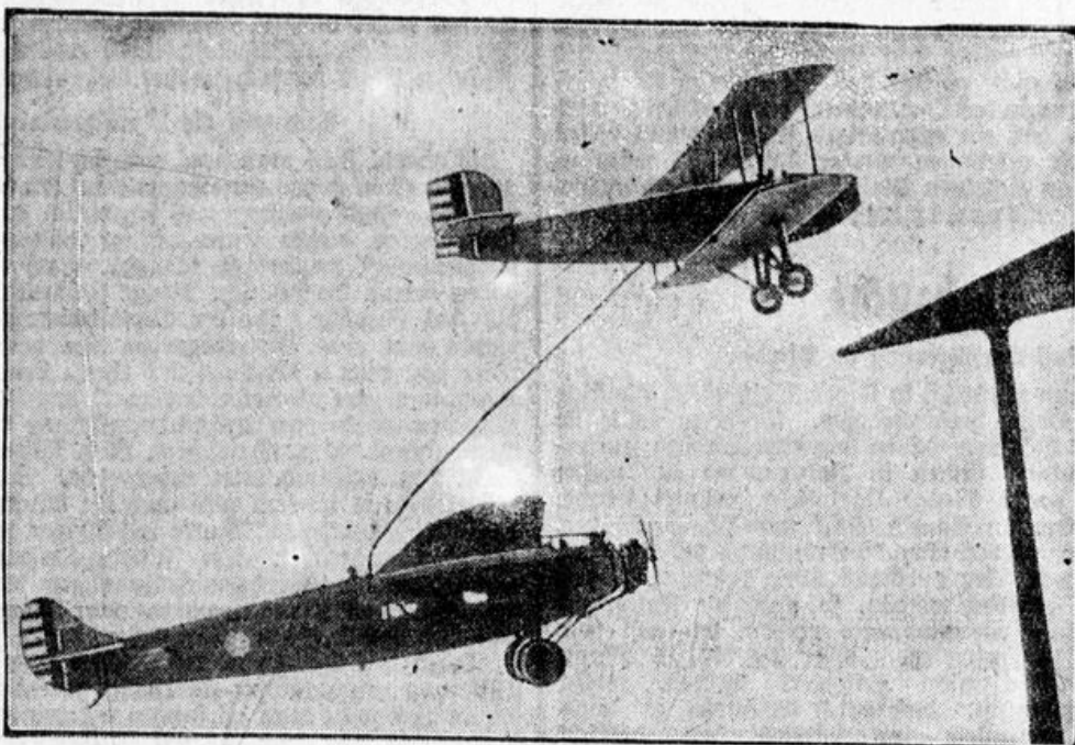
Überführen von Benzin mittels Schlauch von einem Flugzeug zum andern.
