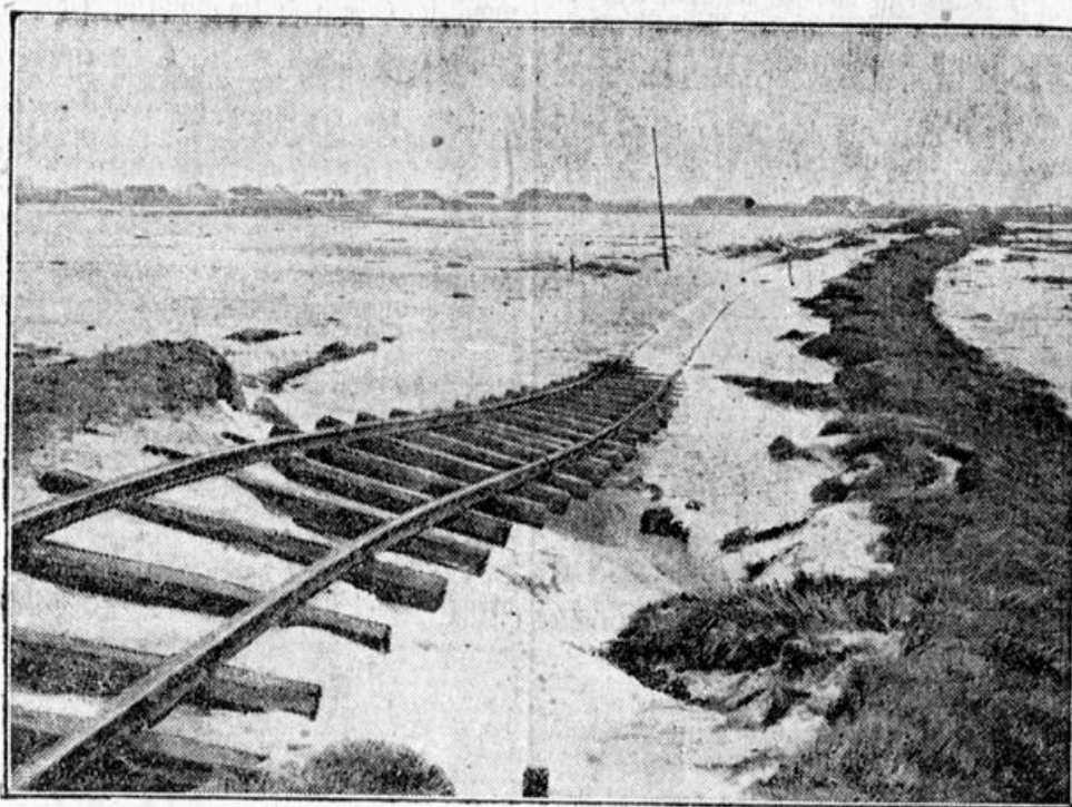
Der zerbrochene Bahndamm der Sylter Eisenbahn bei Hörnum.
