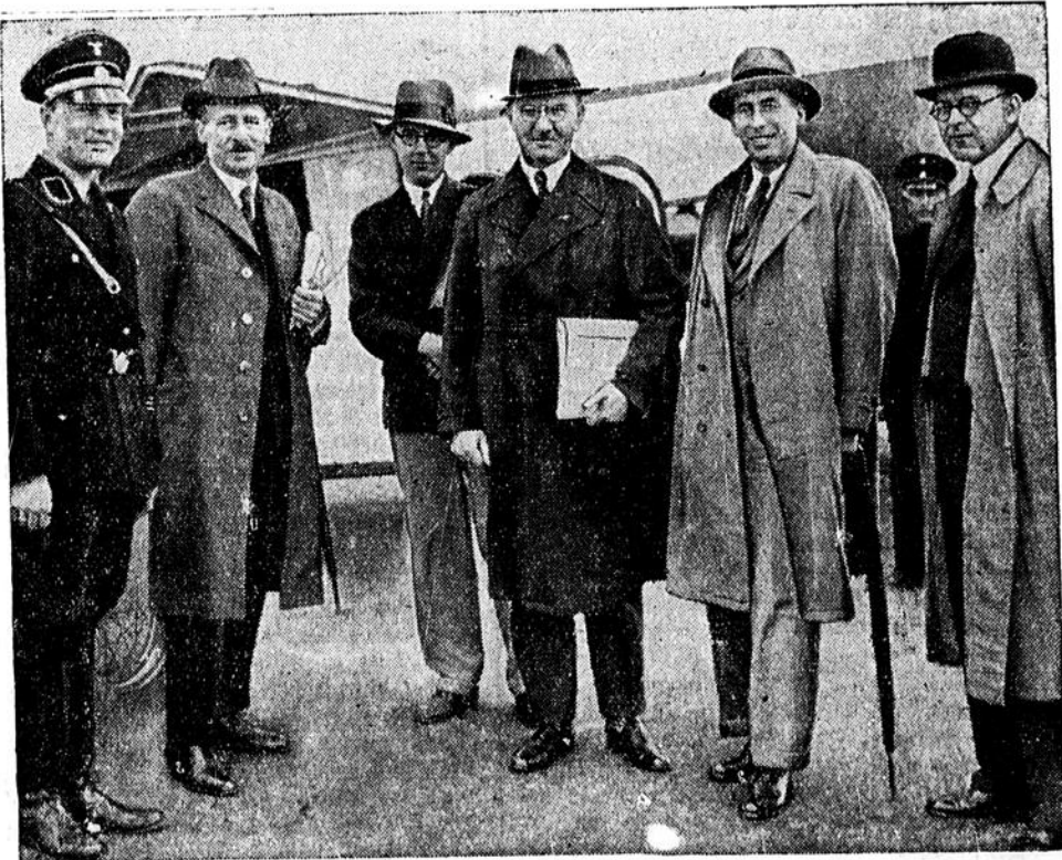
Reichsbankpräsident Schacht zurückgekehrt. Soeben sind der Reichsbankpräsident Schacht (1), der Bürgermeister von Hamburg, Krogmann (2) und der Wirtschafts-
