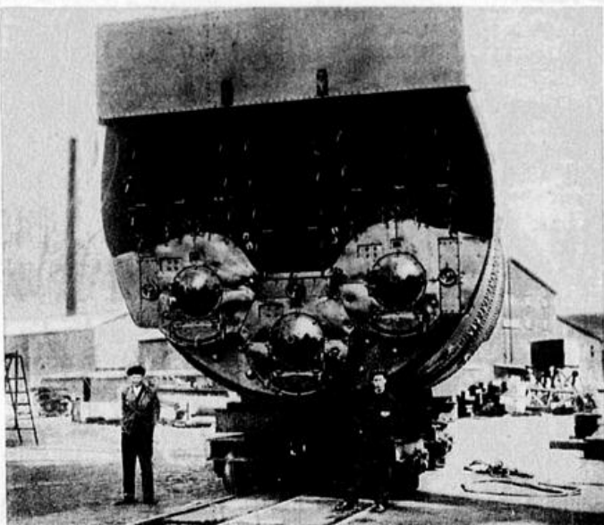
Das Herz des Ozeandampfers. Ein zum Einbau fertiger Kessel für einen modernen Schiffsriesen. Der Vergleich mit den nebenstehenden Personen läßt den gewaltigen Umfang erkennen. Atlantik
