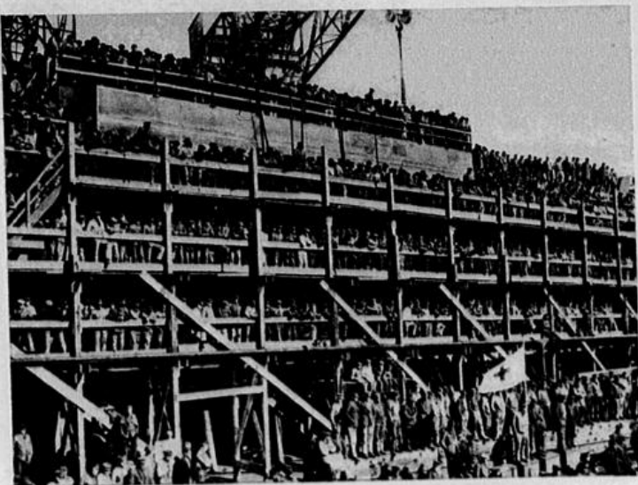
Eine eigenartige Zuschauertribüne in der Wilhelmshavener Werft. Die Werftarbeiter sahen dem Stapellauf der Torpedoboote von einem Gerüst aus zu, das nebenan um ein im Bau begriffenes Schiff errichtet ist Photo-Union
