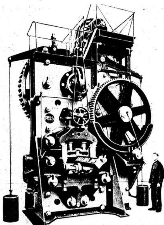
Eine Riesenblockschere aus der Erfurter Maschinenfabrik, die Eisenplatten im Durchmesser von 21 cm auf kaltem Wege mit einem einzigen Hieb durchschneidet
